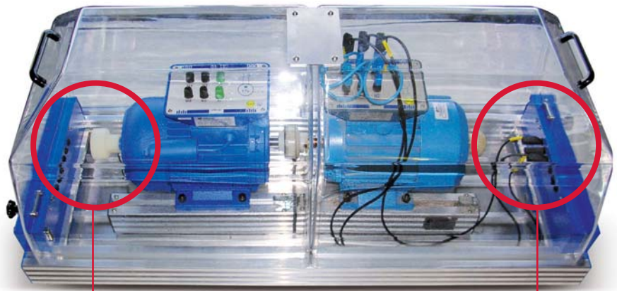
Guardas de protección y enclavamientos mecánicos
